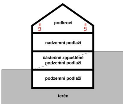
Vzorový řez
